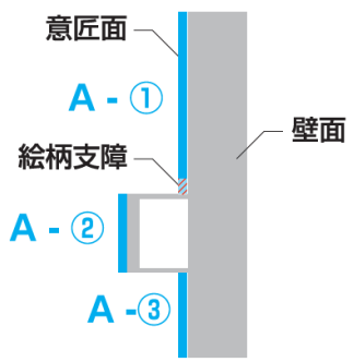
断面図
